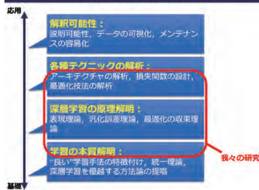
深層学習の理論概観
